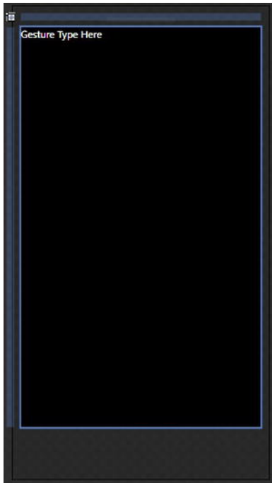
Figure 8-15. UIElementRenderer Xaml
