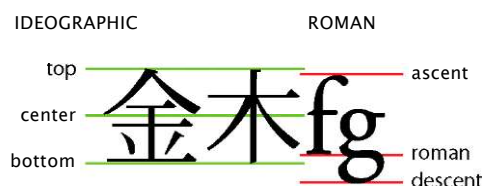
Figure 10-9. TLF text baselines
